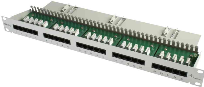
19" ISDN Patch Panel mit Adernmanagement
