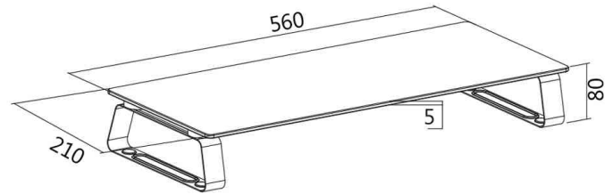
Monitorständer - Abmessungen
