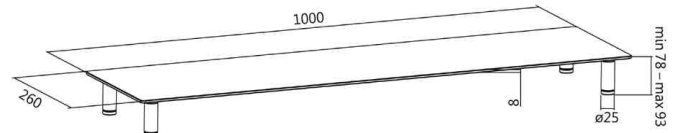
Monitorständer, extra breit - Abmessungen
